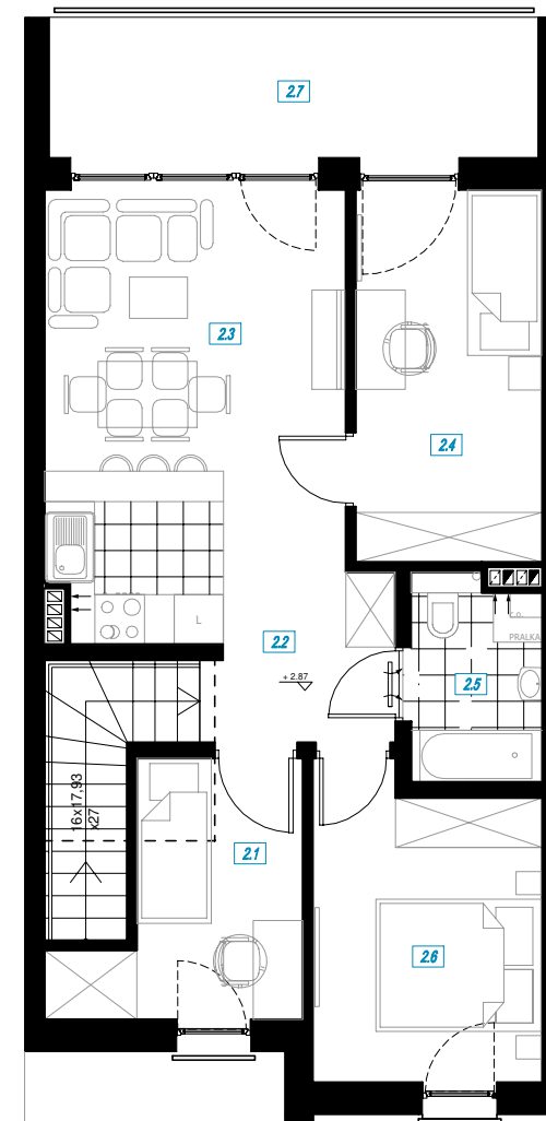
PIĘTRO
